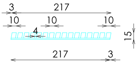
ALZADO
