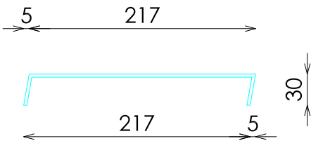
ALZADO
