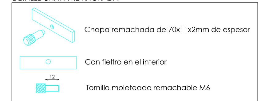
DETALLE ANCLAJE
