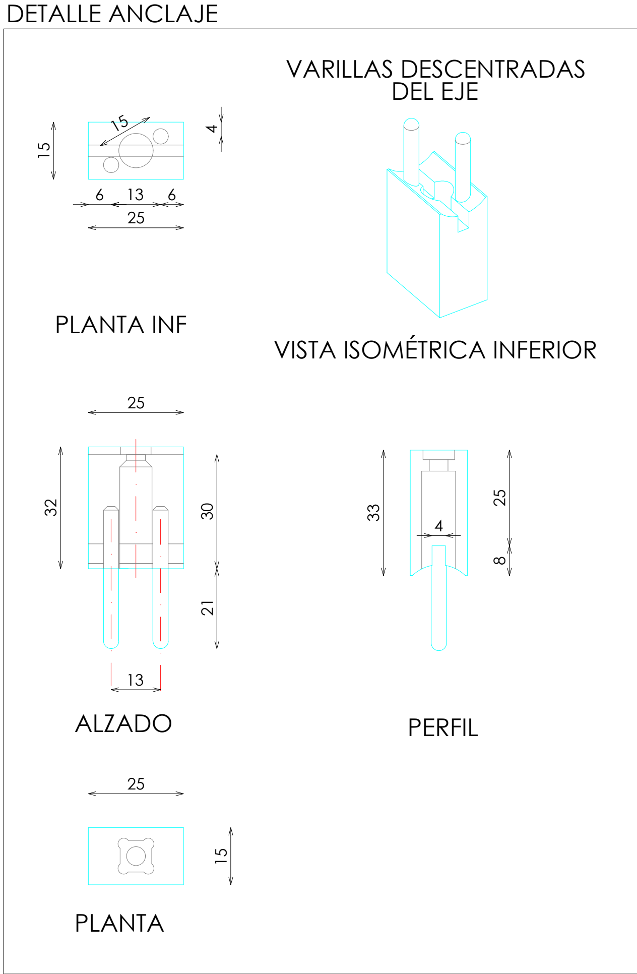
DETALLE ANCLAJE
