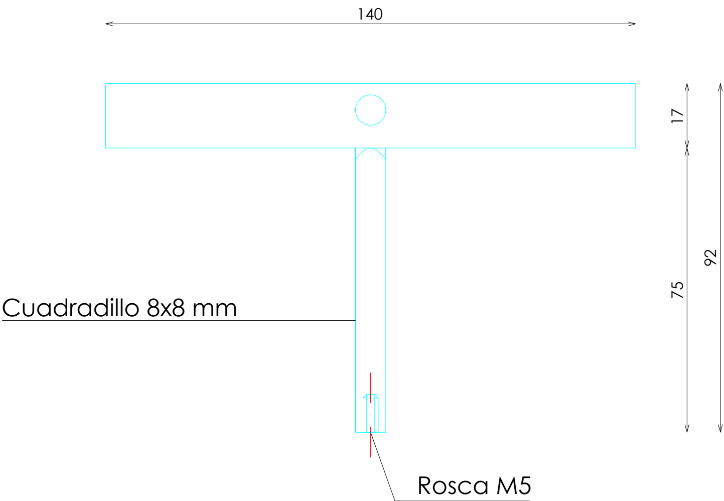
ALZADO
