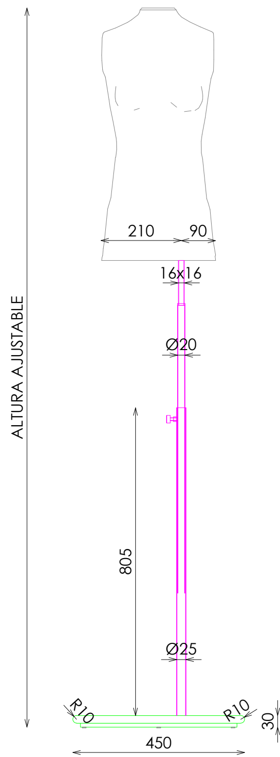
ALZADO
