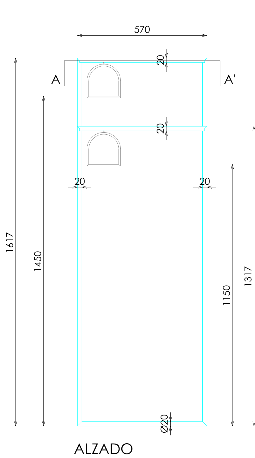
ALZADO
