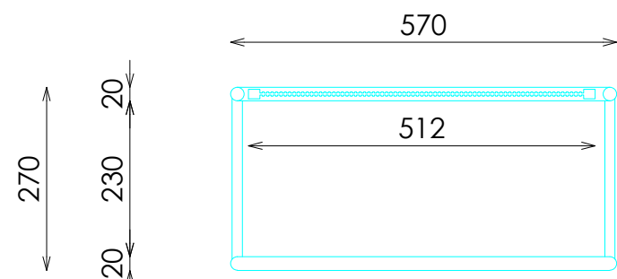
SECCIÓN AA'
