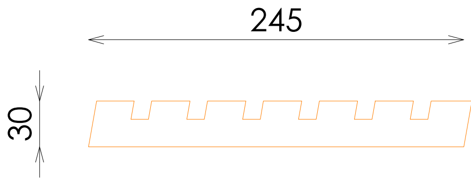
ALZADO
