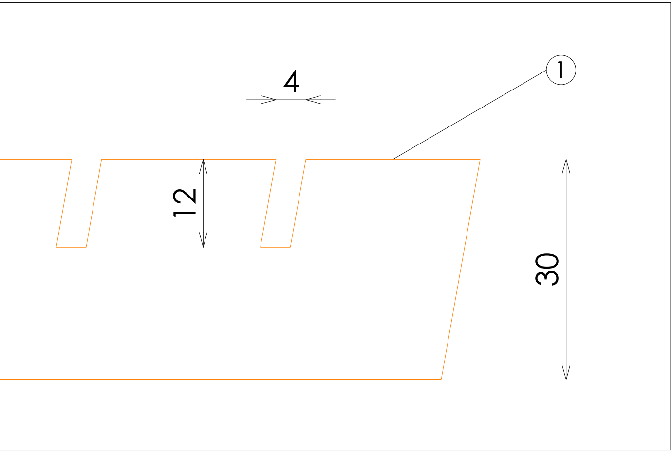
DETALLE BANDEJA
