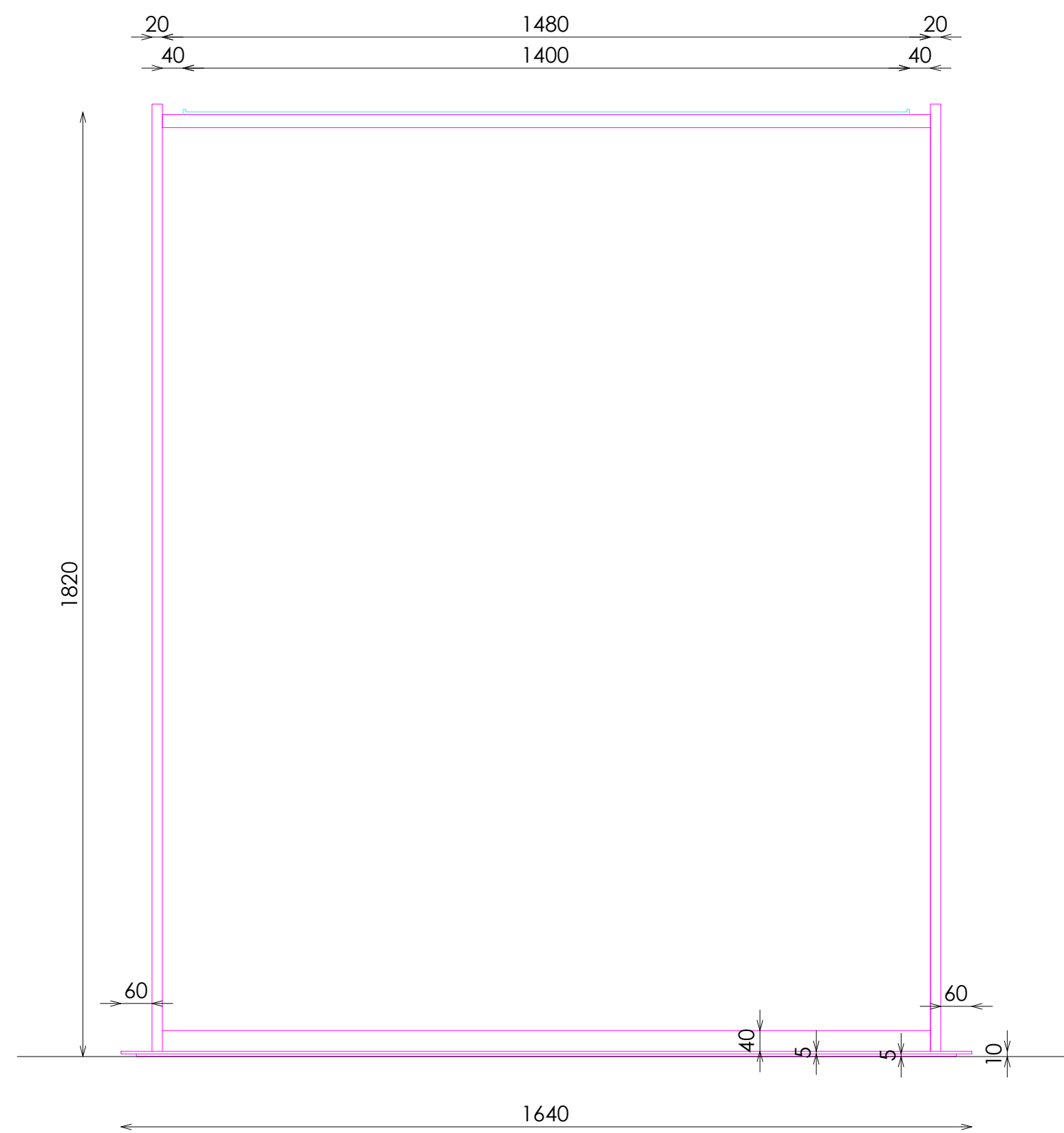
ALZADO SECCIONADO
