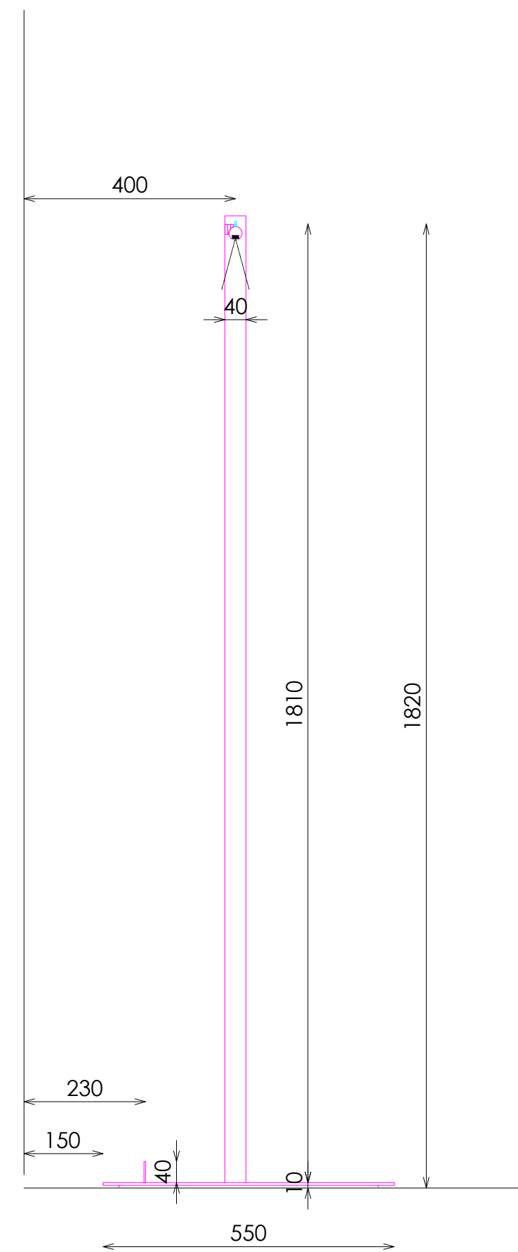
PERFIL SECCIONADO
