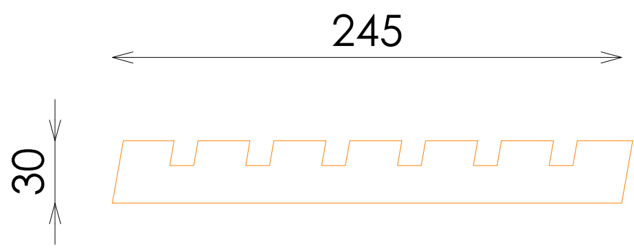
ALZADO RANURA 11
