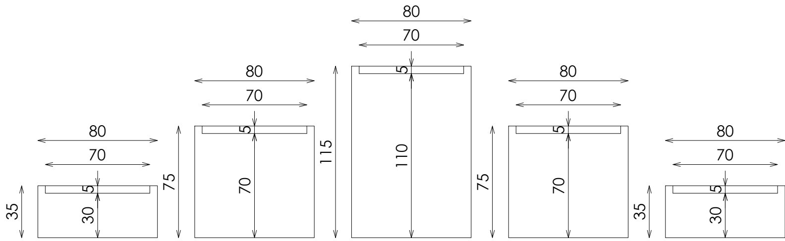
SECCION
