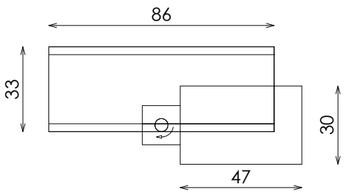
PLANTA POSICION 1
