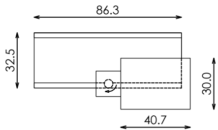
PLANTA POSICION 1
