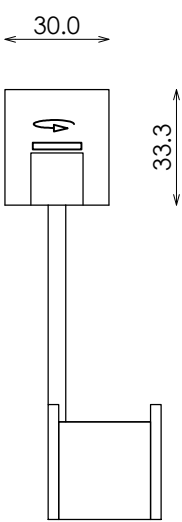
ALZADO
