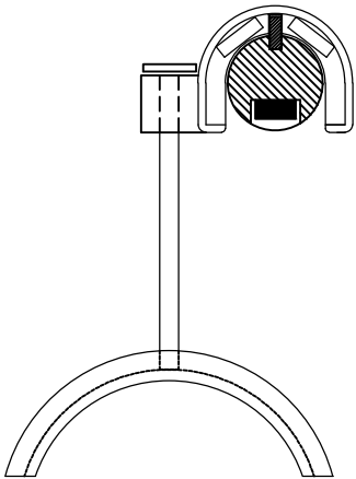
DETALLE MONTAJE POSICION 1
