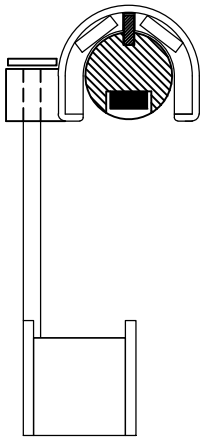
DETALLE MONTAJE POSICION 2
