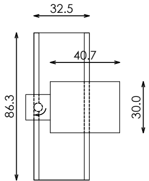
PLANTA POSICION 2
