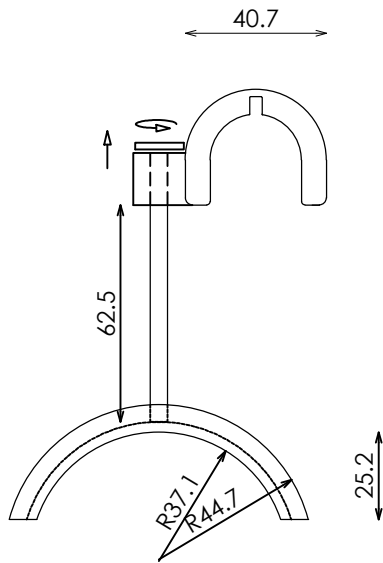
ALZADO
