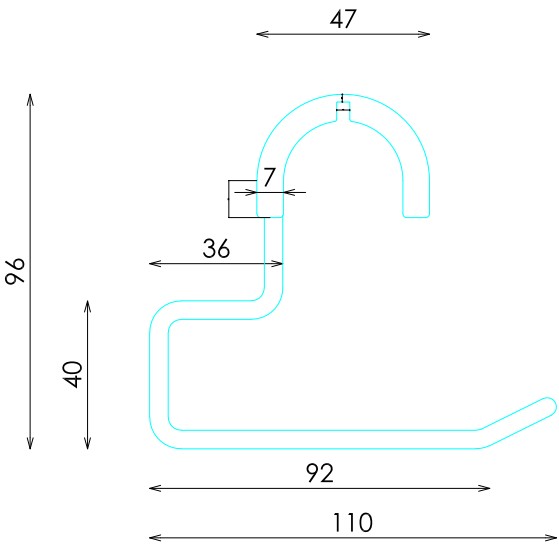
ALZADO
