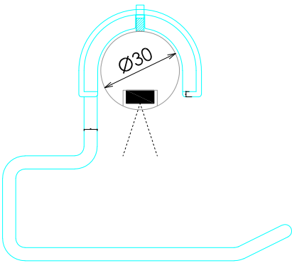
DETALLE MONTAJE BARRA Ø30
