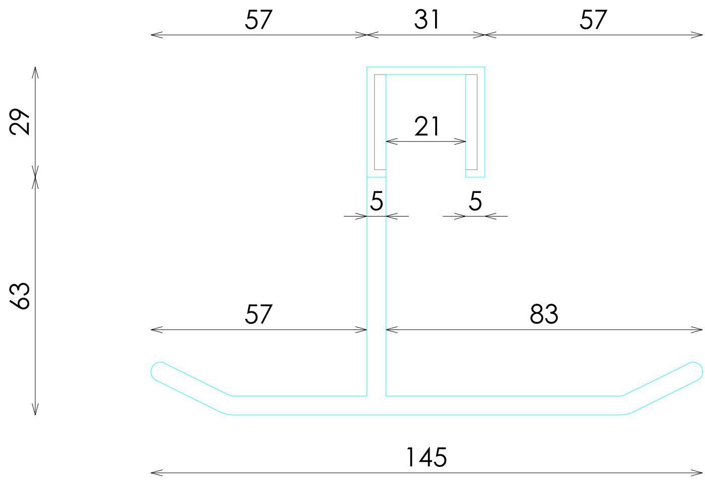
ALZADO
