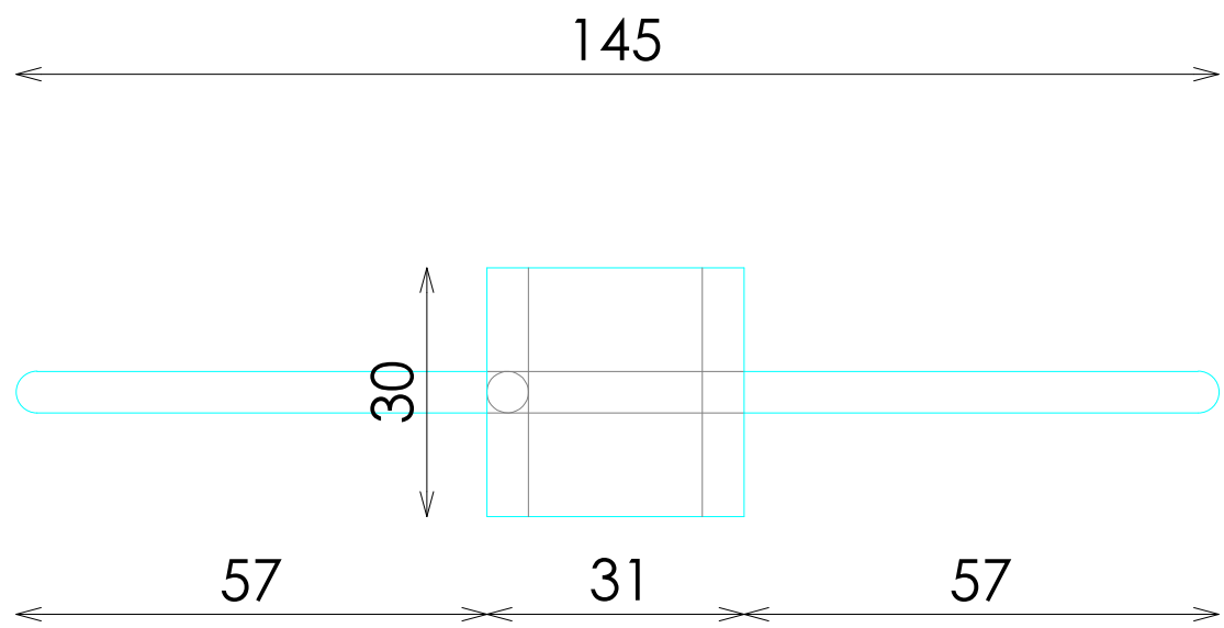
PLANTA
