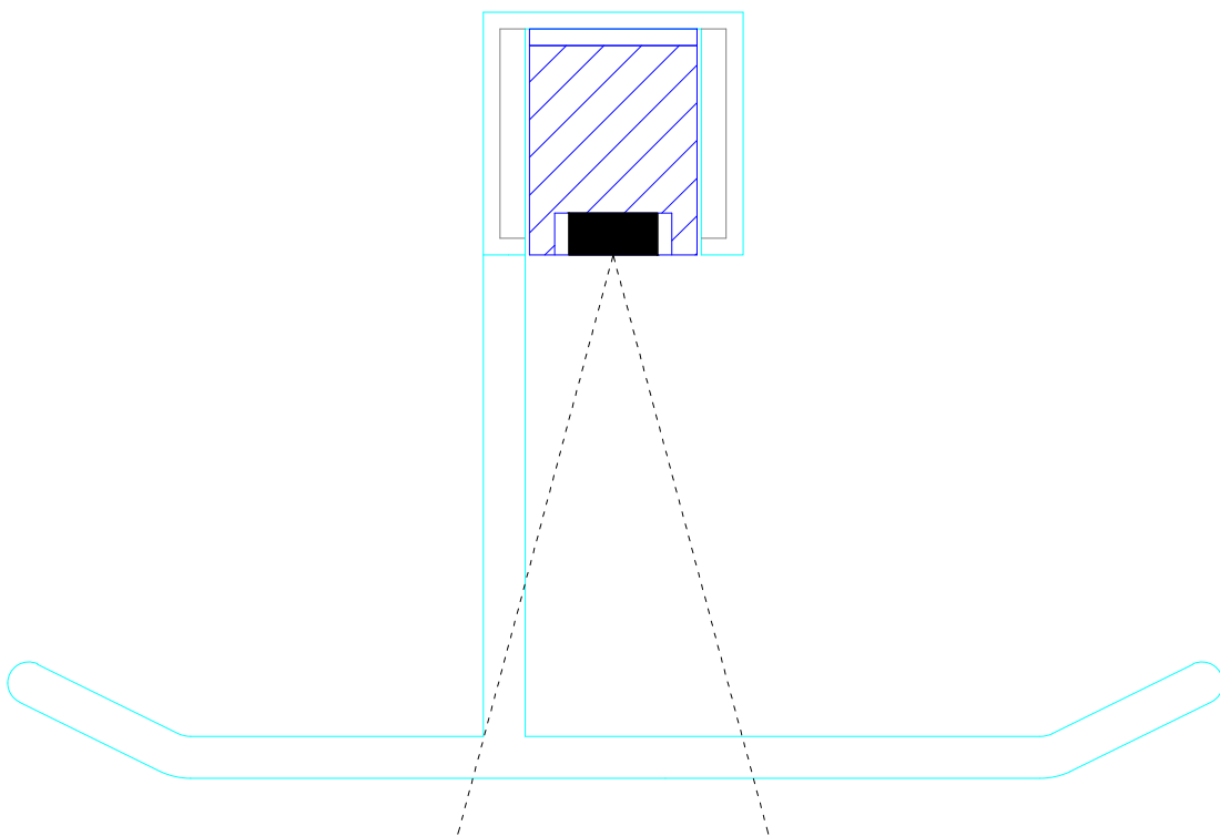
SECCION MONTAJE BARRA 20x25
