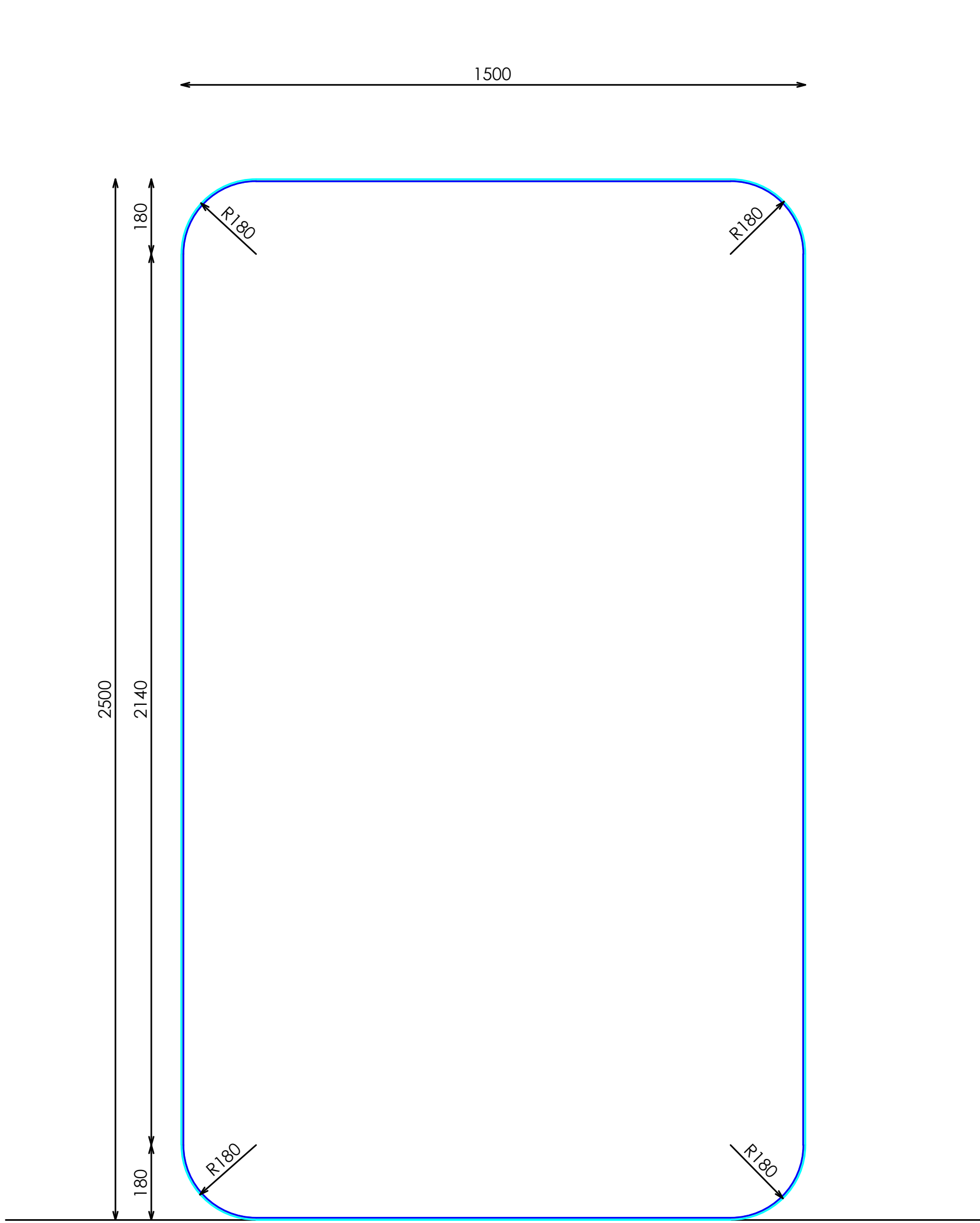
ALZADO
