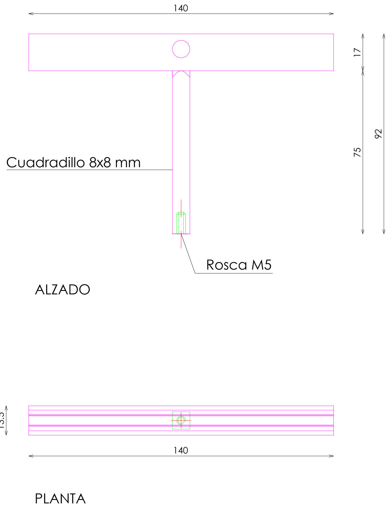
PLANTA
