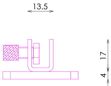
PERFIL
