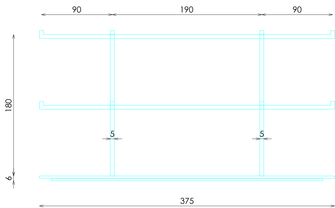
ALZADO
