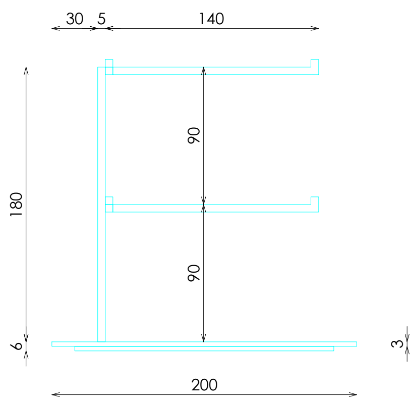
PERFIL
