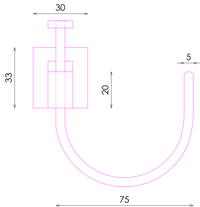
ALZADO
