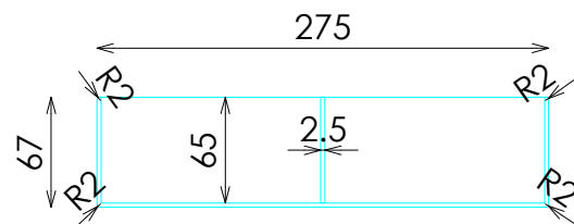
SECCION LONGITUDINAL
