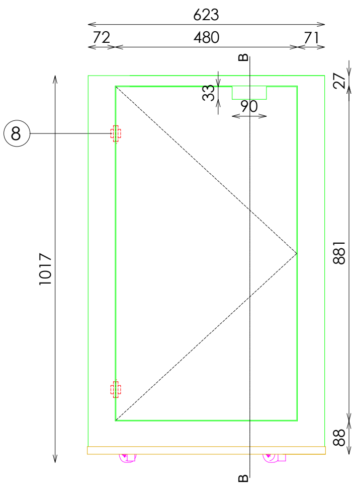
ALZADO
