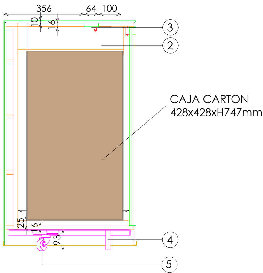
SECCION B-B
