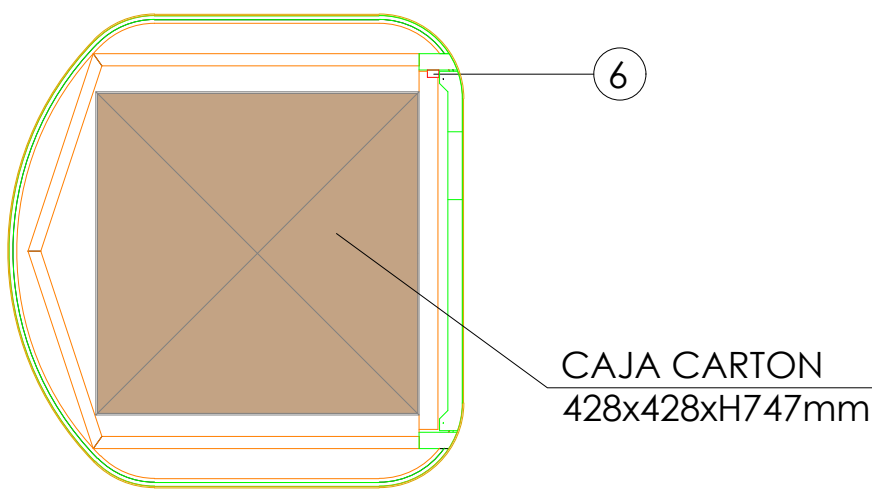
SECCION A-A
