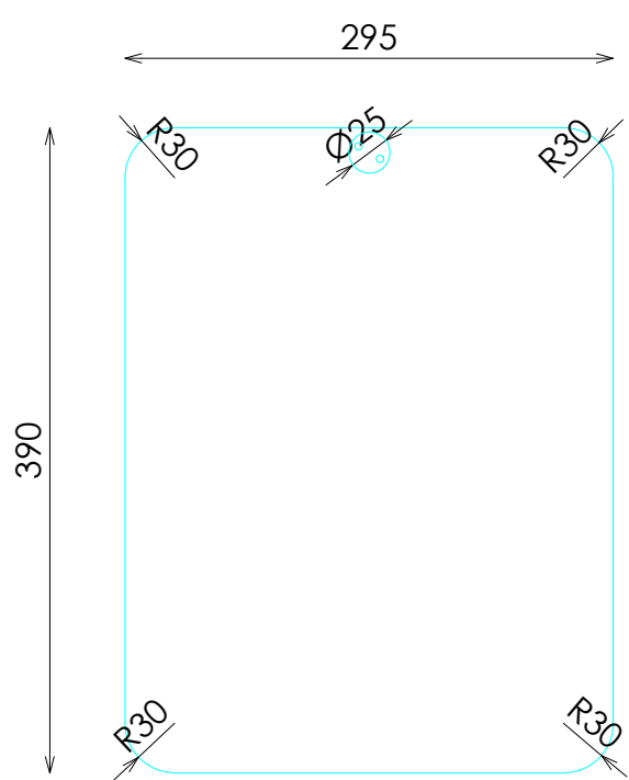
PLANTA
