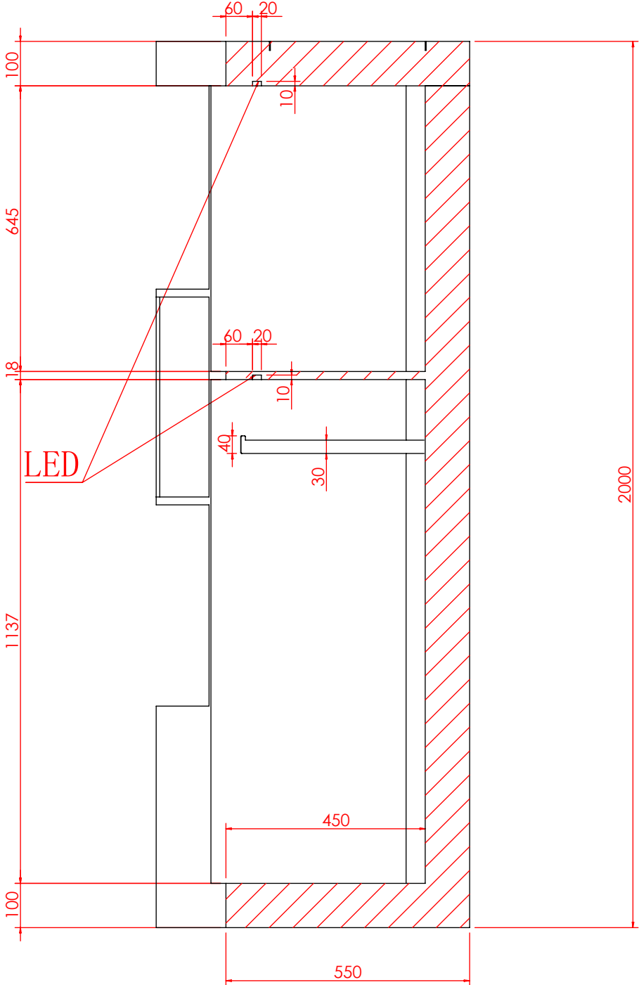
剖面 AW-AW
