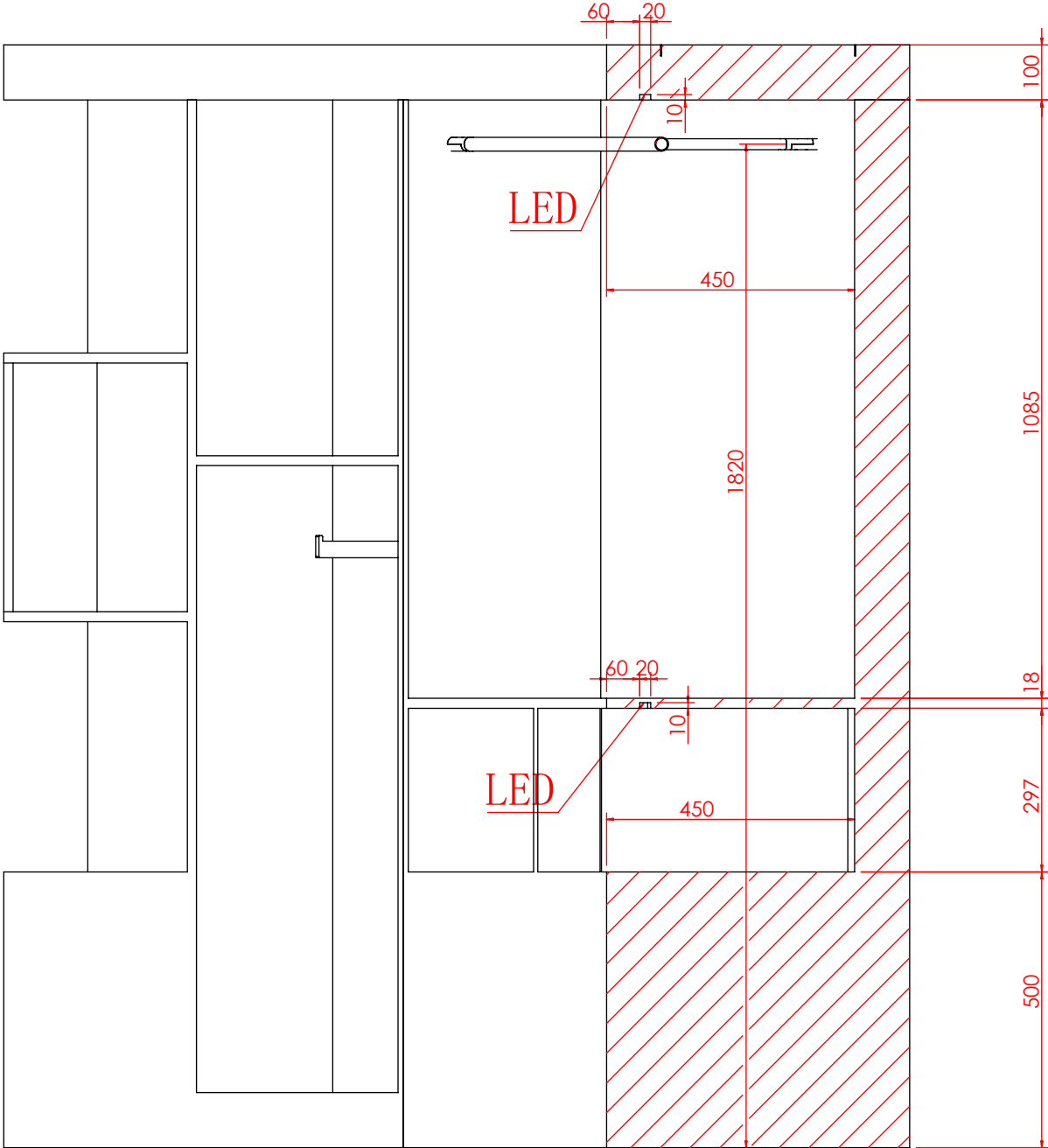
剖面 AV-AV
