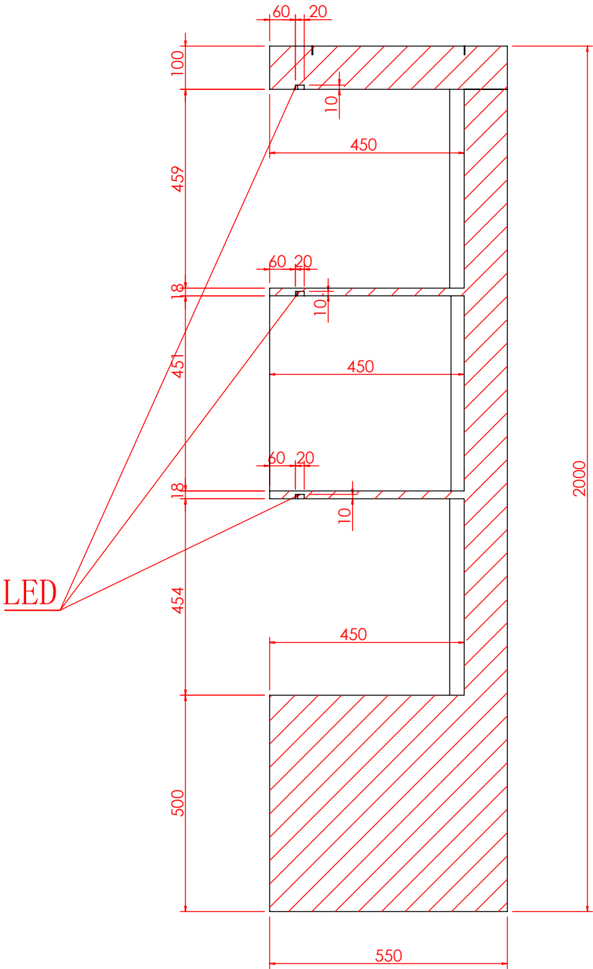
剖面 AX-AX
