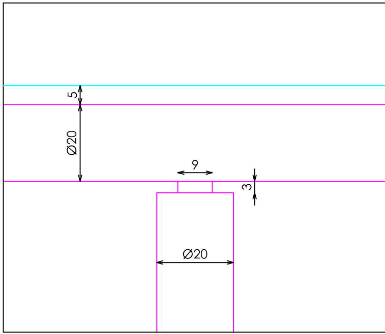
DETALLE A
