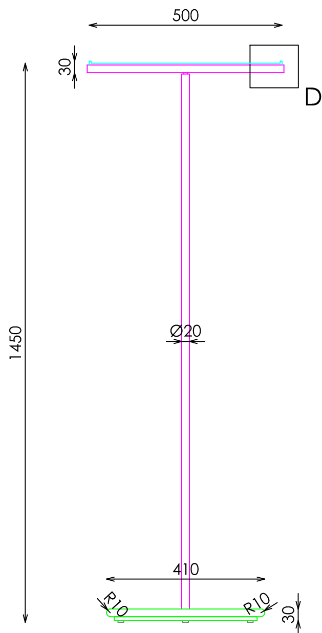
ALZADO
