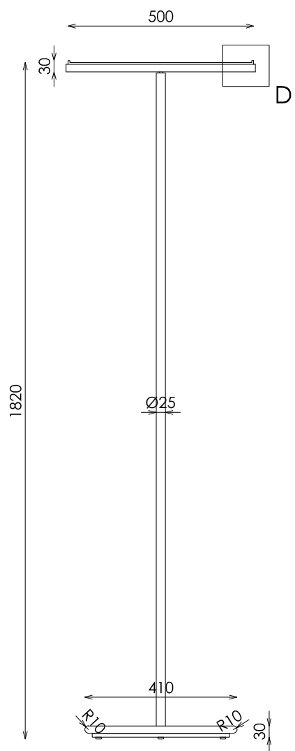
ALZADO
