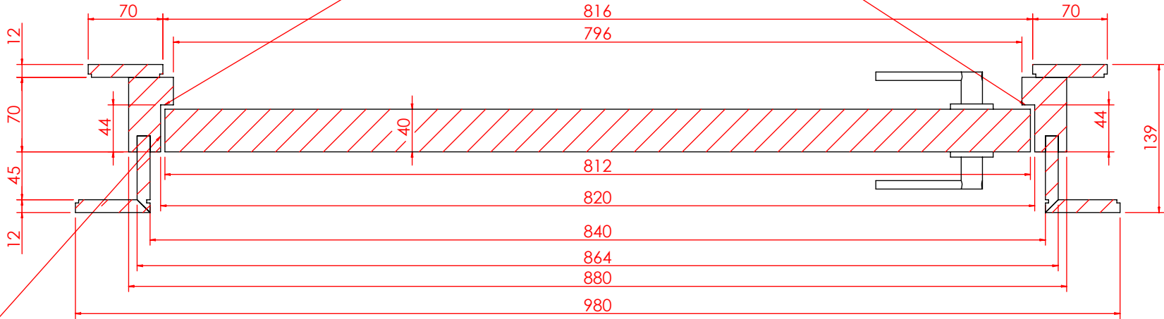
剖面 AG-AG 比例 1:5
