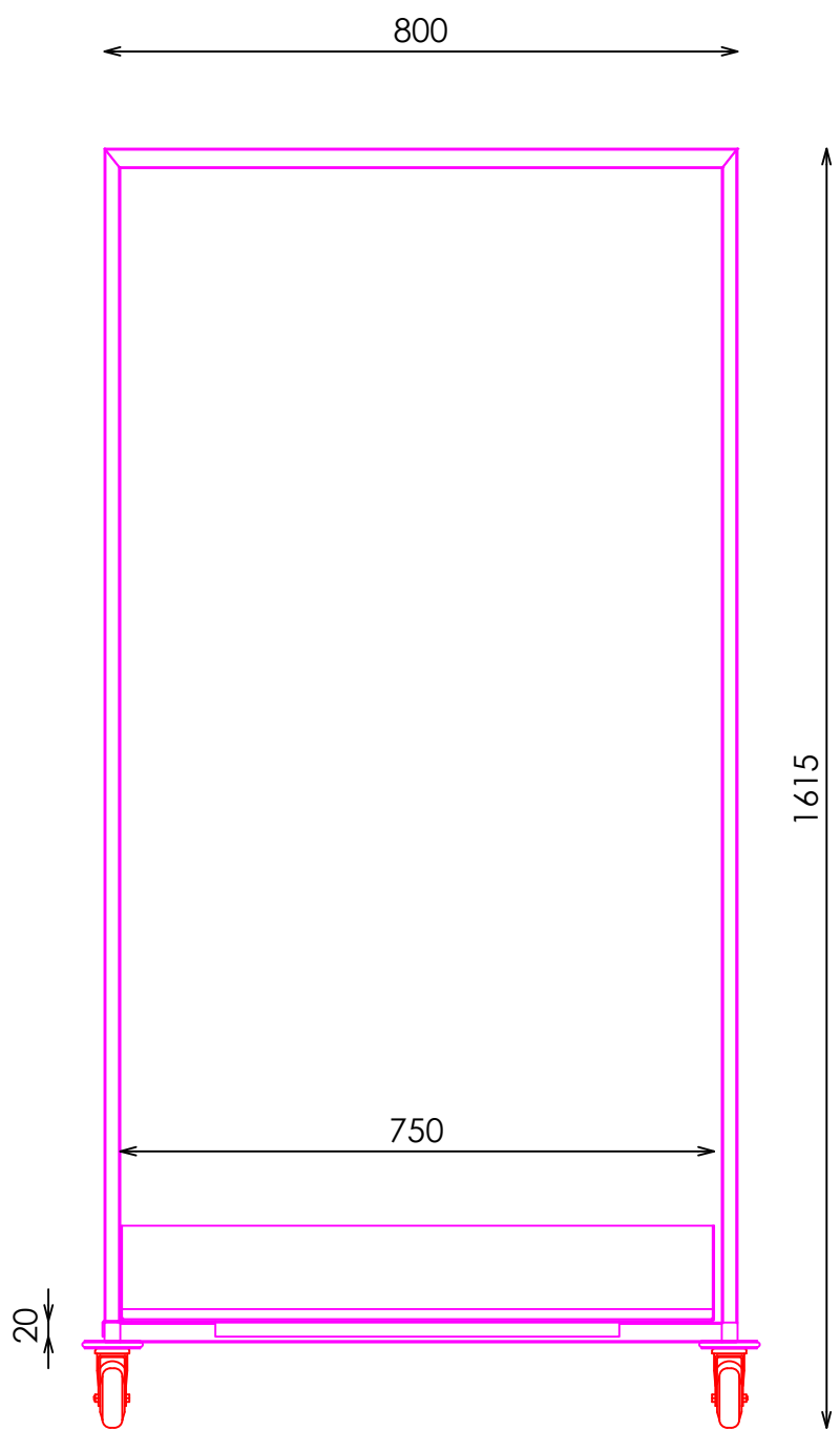
ALZADO FRONTAL
