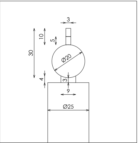
DETALLE B
