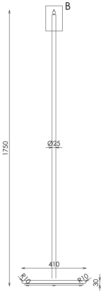
PERFIL
