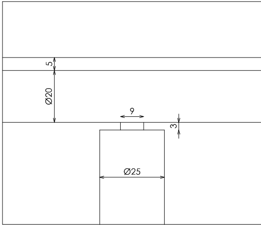
DETALLE A
