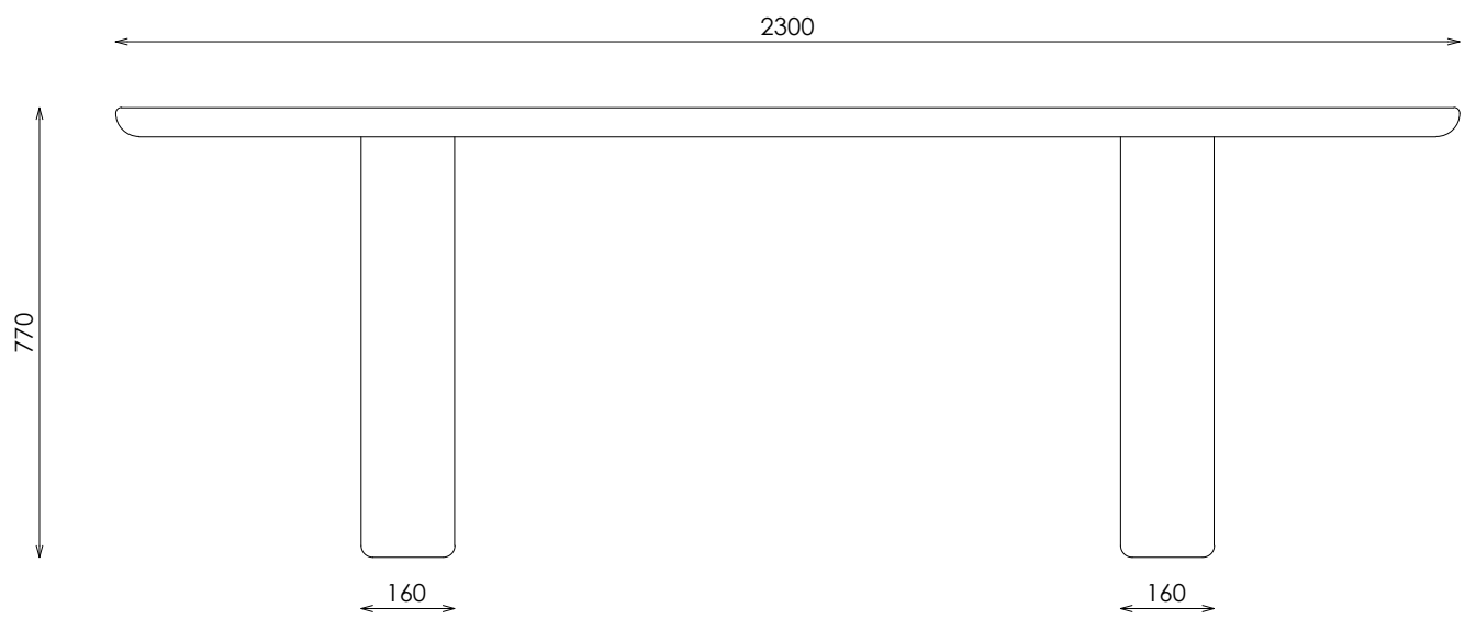
ALZADO FRONTAL
