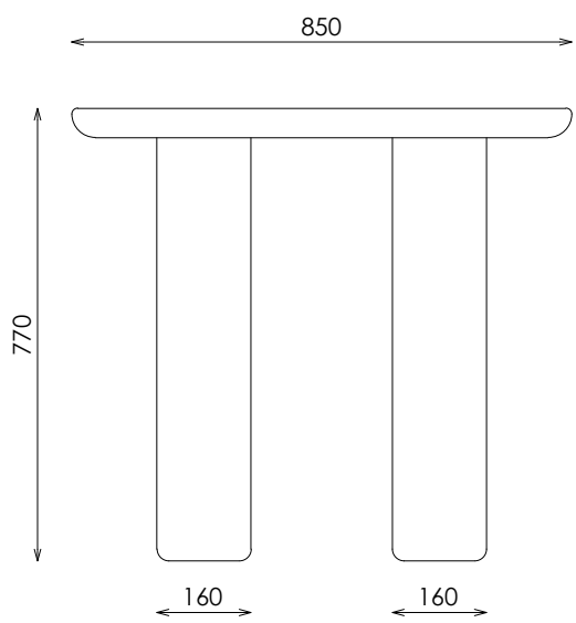
ALZADO LATERAL
