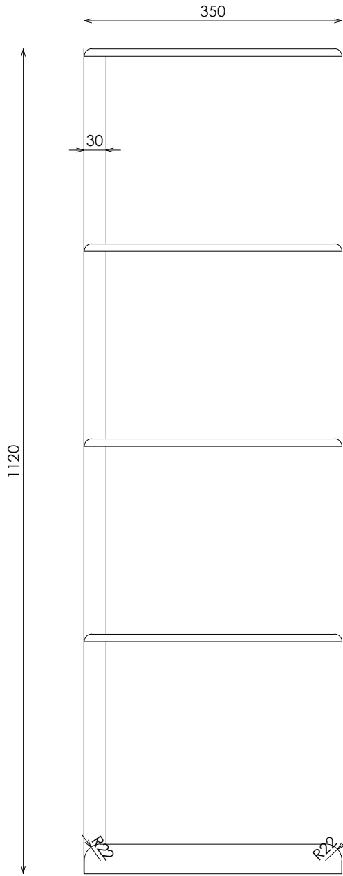
ALZADO LATERAL
