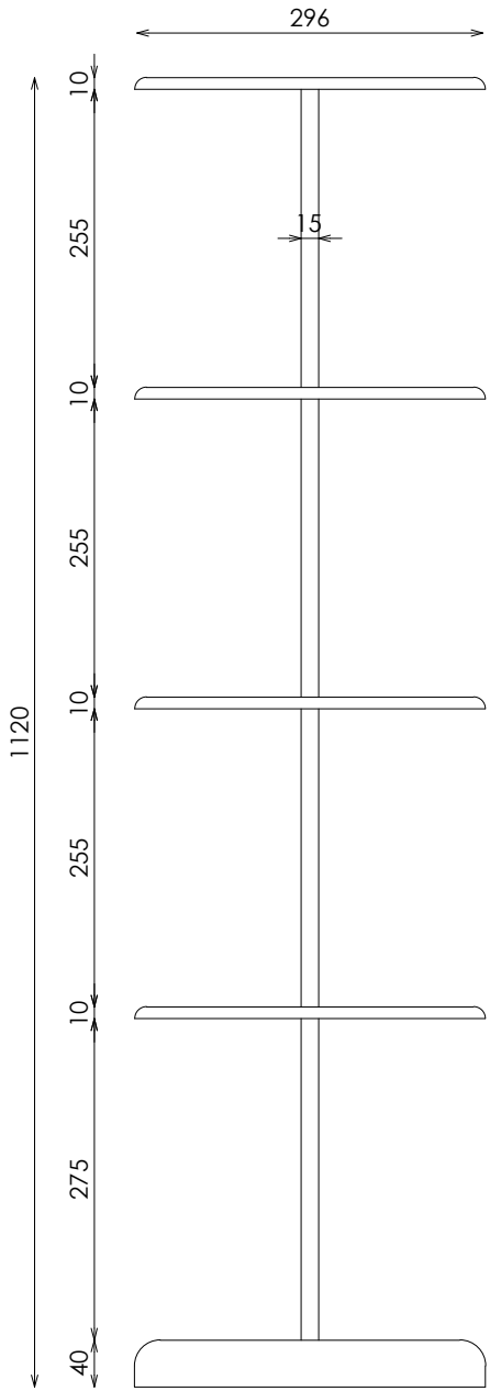
ALZADO
