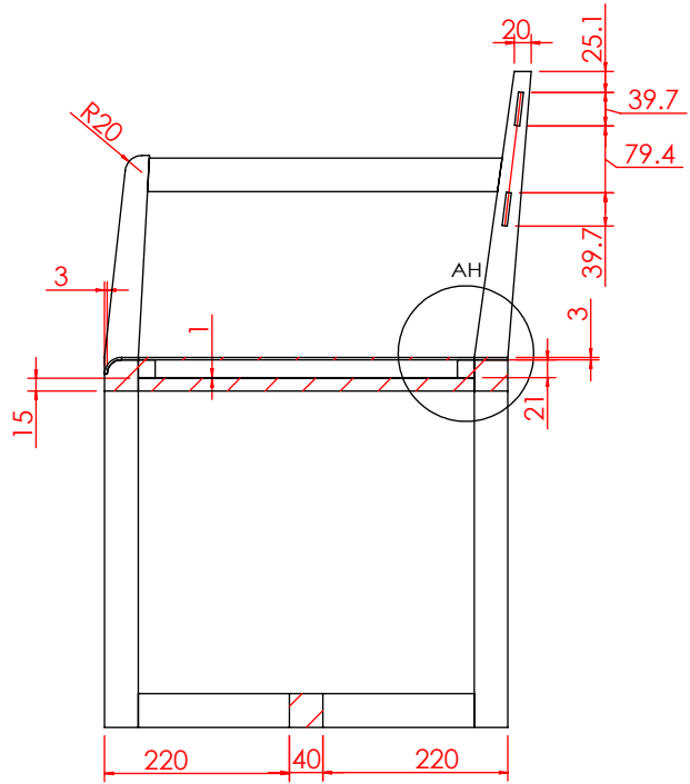
剖面 AG-AG
