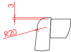
局部视图 AM 比例 1 : 5
