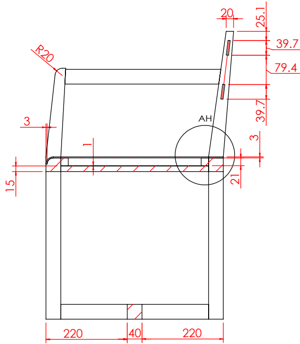
剖面 AG-AG
