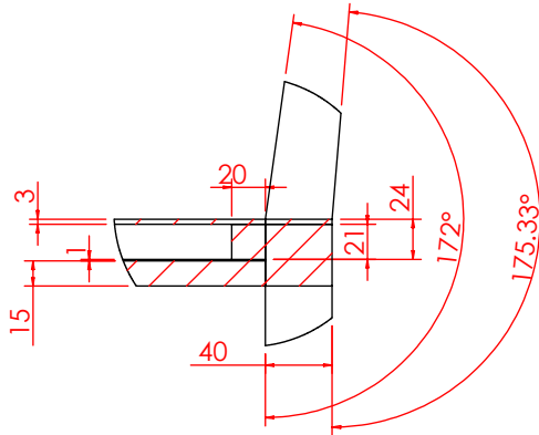
局部视图 AH 比例 1 : 5
