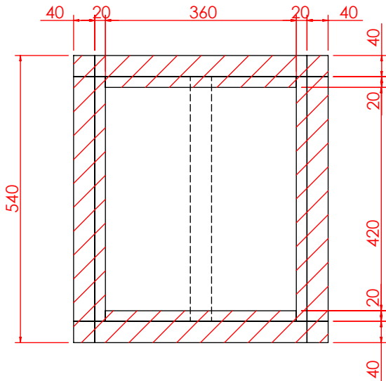
剖面 AK-AK
