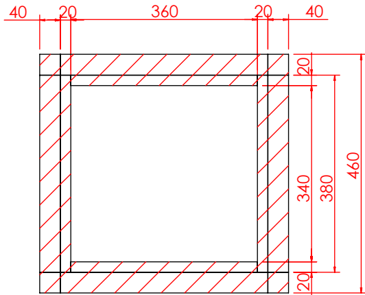
剖面 AK-AK
