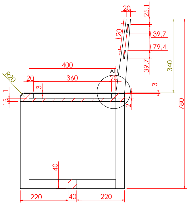
剖面 AG-AG
