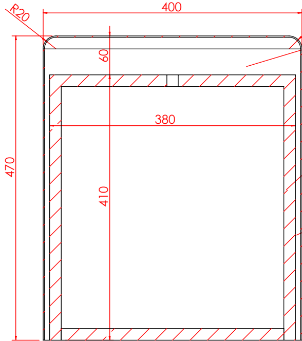
剖面 AG-AG
