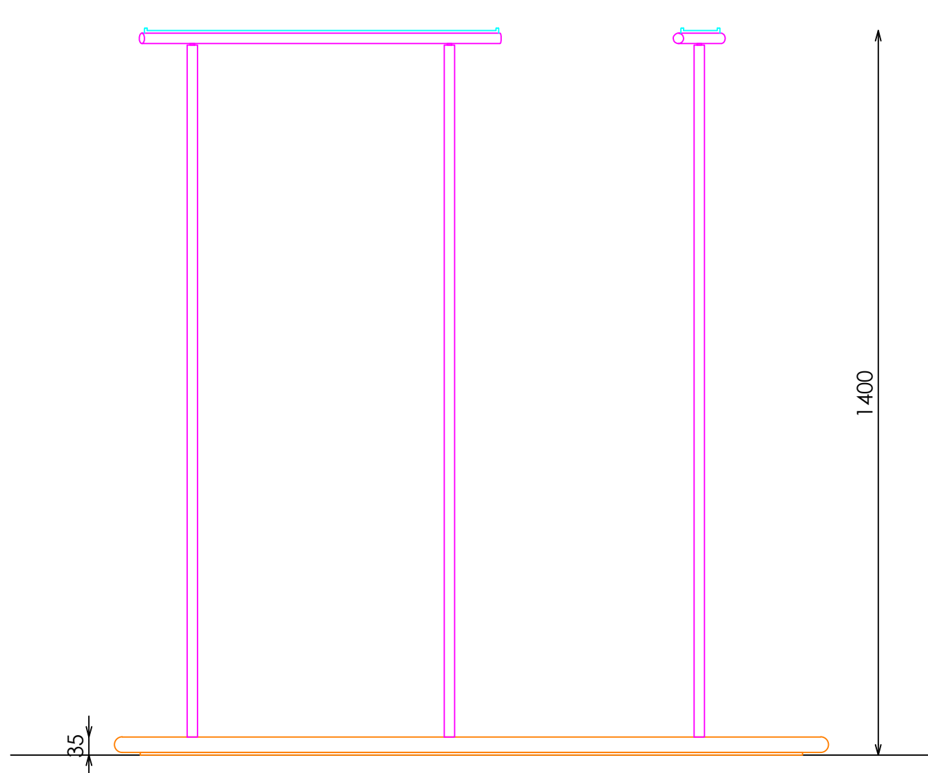
ALZADO FRONTAL
