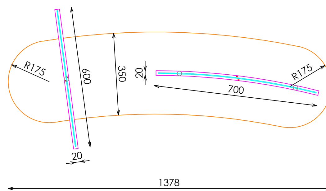
PLANTA
