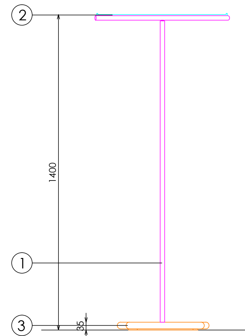
ALZADO LATERAL
