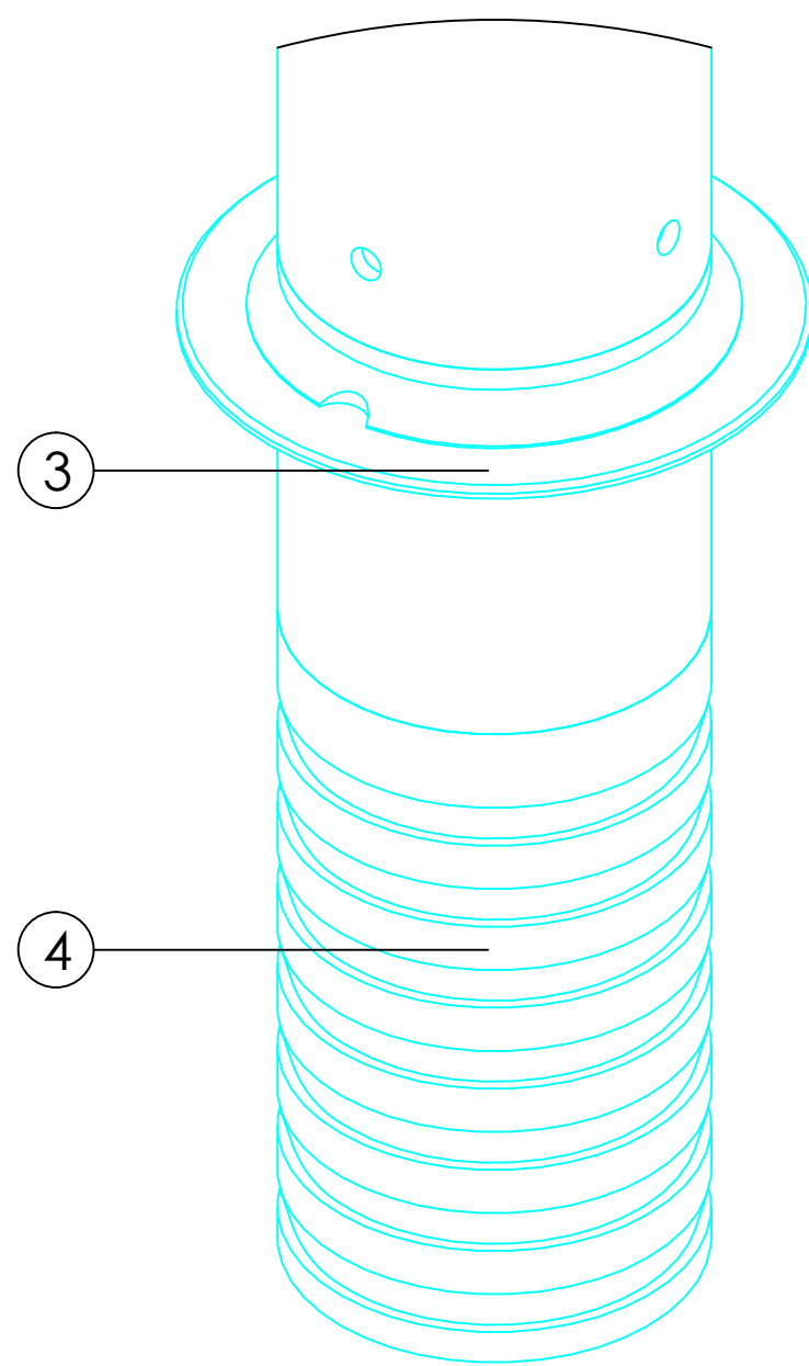
CASQUILLO FIJACIÓN POSTE-SUELO
