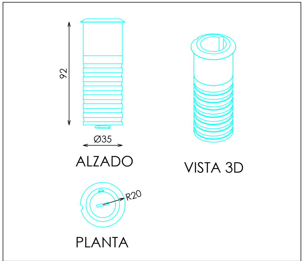
CASQUILLO FIJACIÓN POSTE-SUELO
