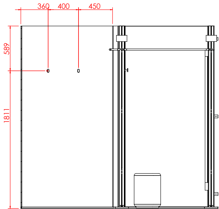
剖面 AG-AG
