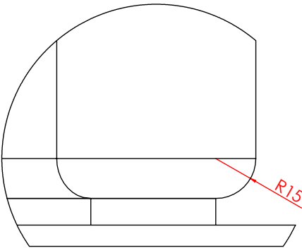
局部视图 AH 比例 1 : 2
