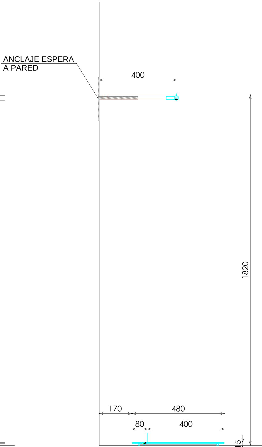
PERFIL SECCIONADO
