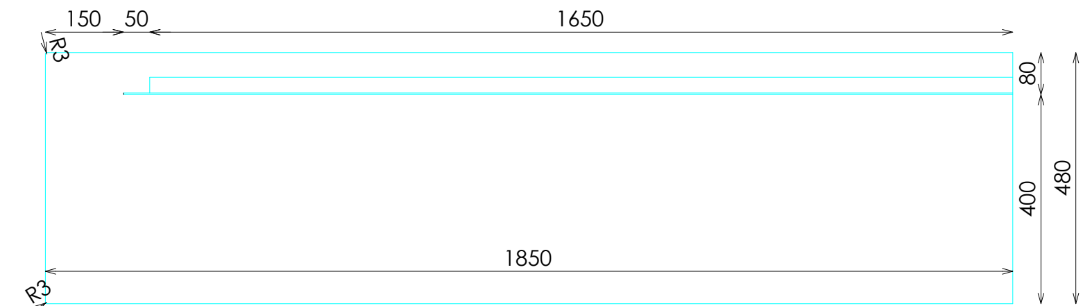
PLANTA TARIMA
