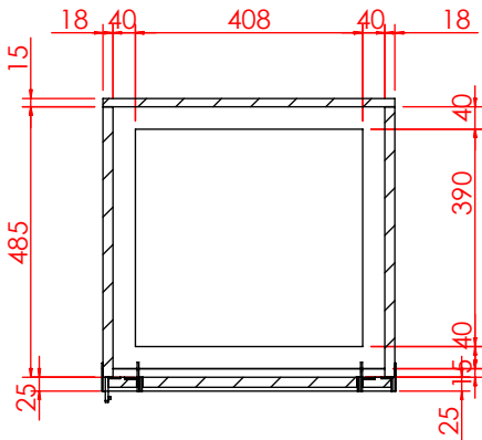
剖面 AH-AH
