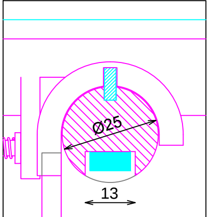
DETALLE ANCLAJE PINCHO COMP.
