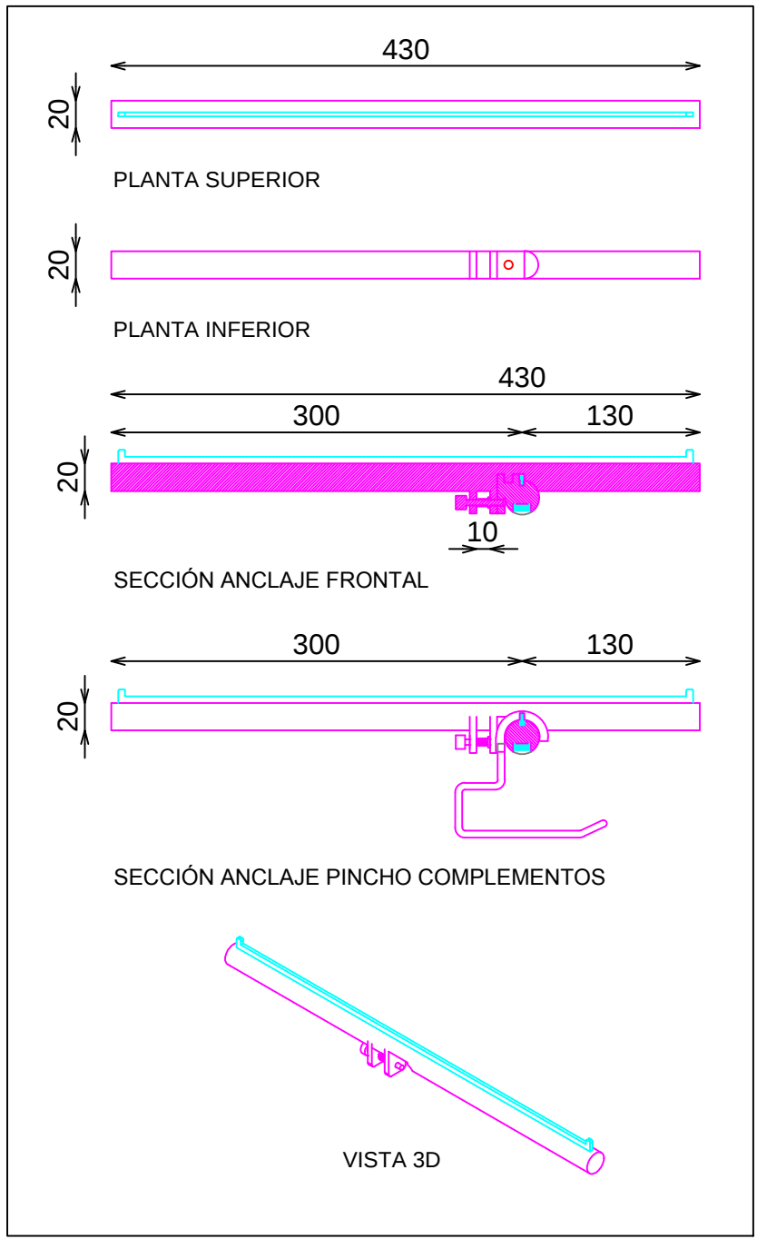
DETALLE ANCLAJE PINCHO COMP.
