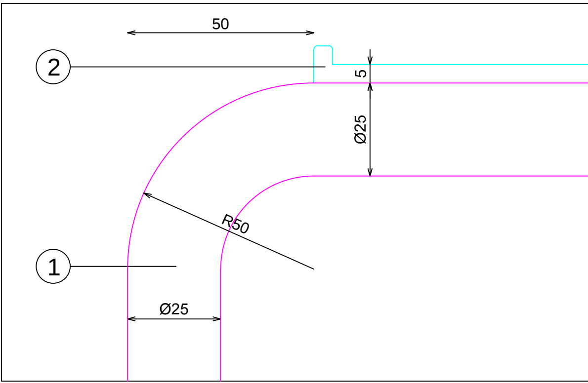
DETALLE ANCLAJE FRONTALES EXTRAIBLES
