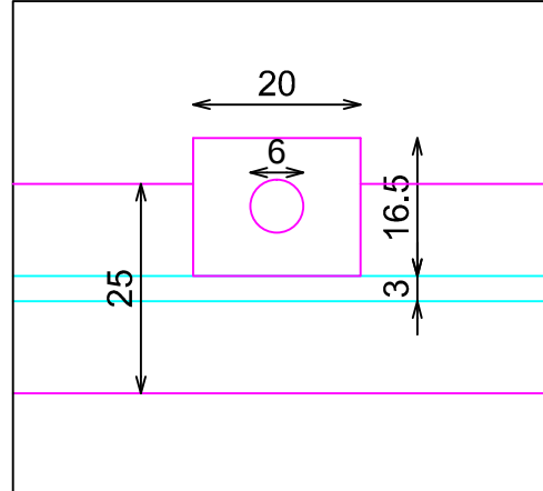
DETALLE BARRA ANCLAJE FRONTALES
