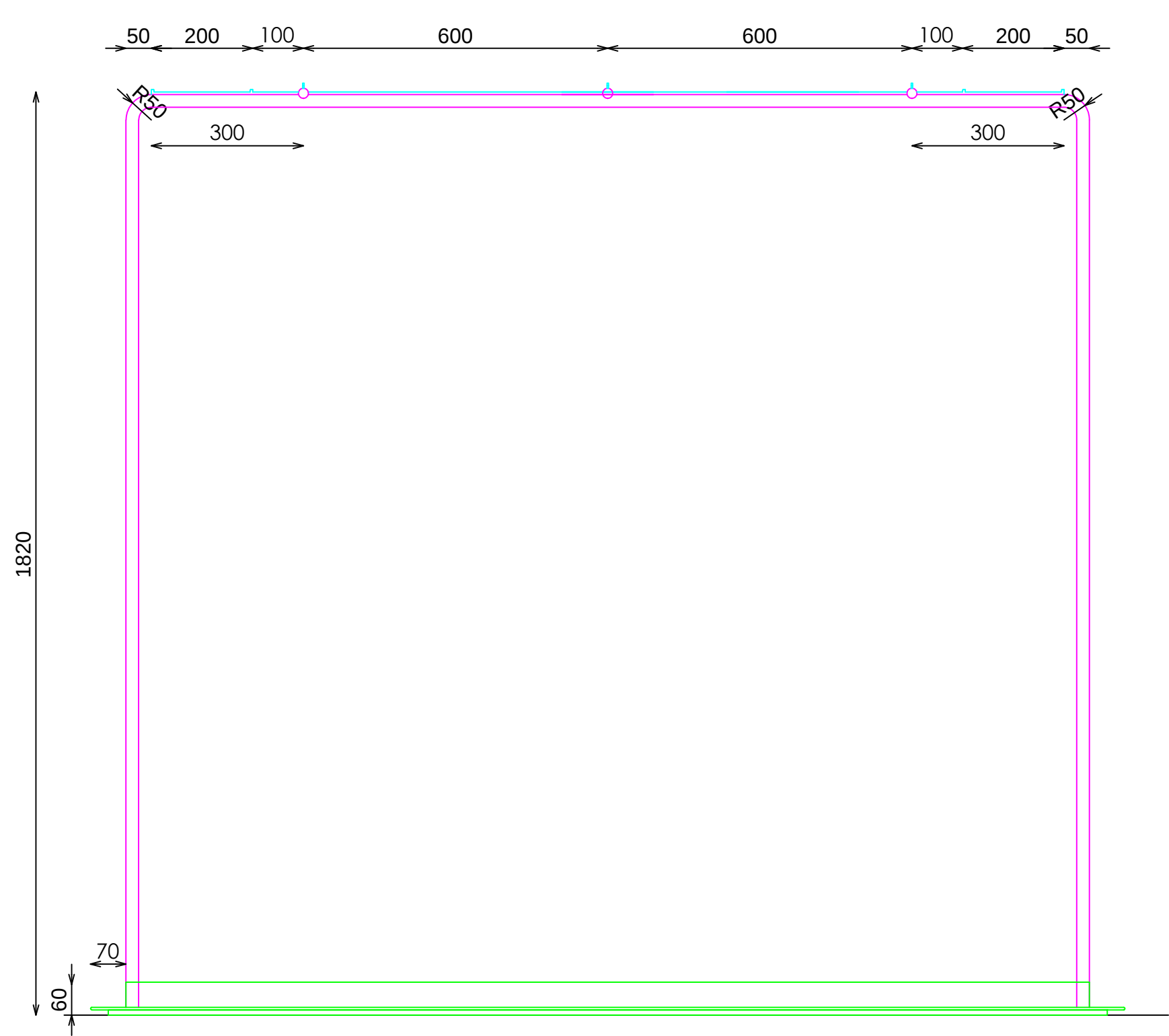
ALZADO FRONTAL
