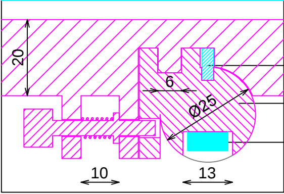
DETALLE ANCLAJE FRONTALES EXTRAIBLES
