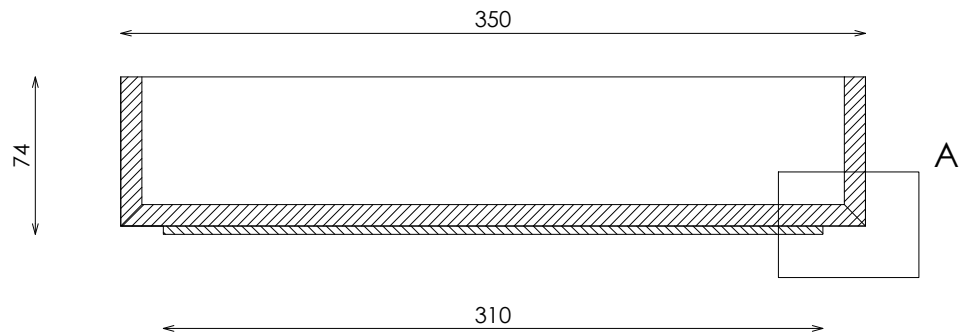
SECCION
