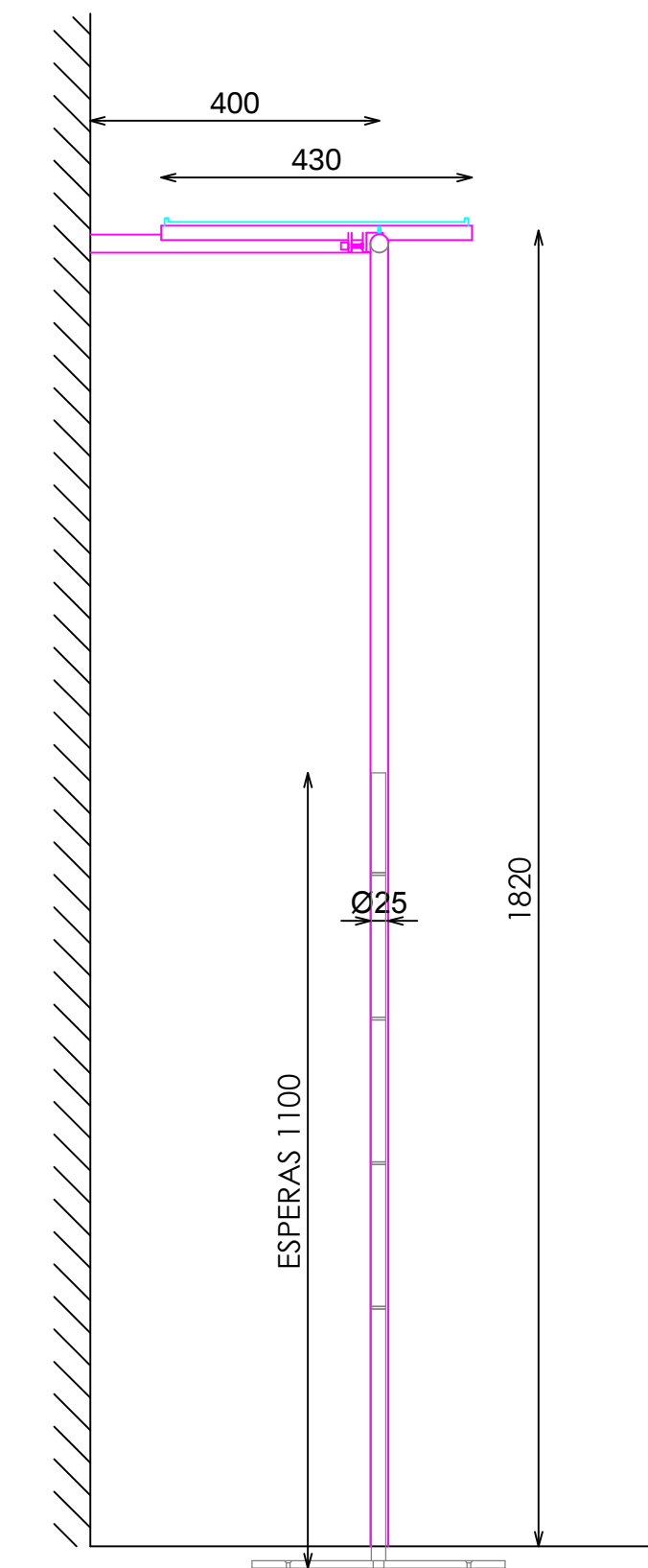
SECCION
