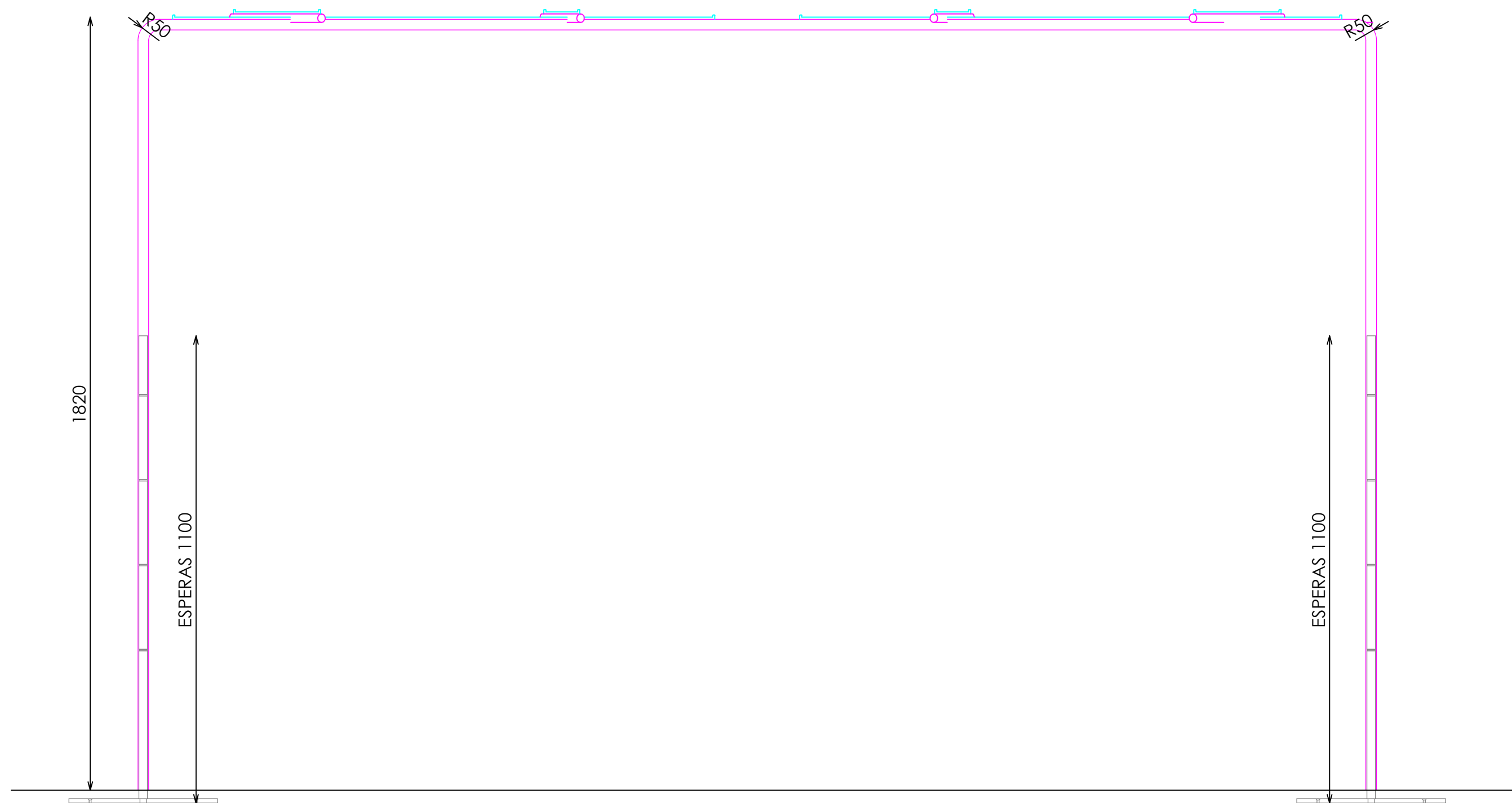
ALZADO FRONTAL
