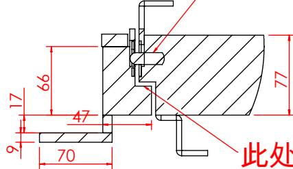
局部视图 AJ 比例 1 : 5
