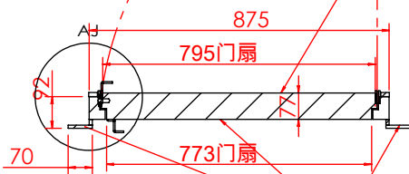
剖面 AI-AJ
