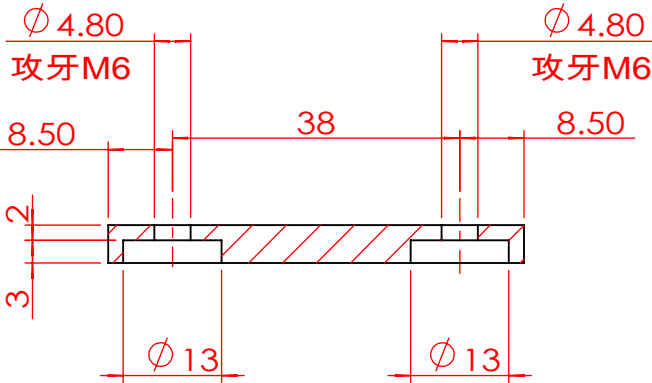
剖面 C-C
