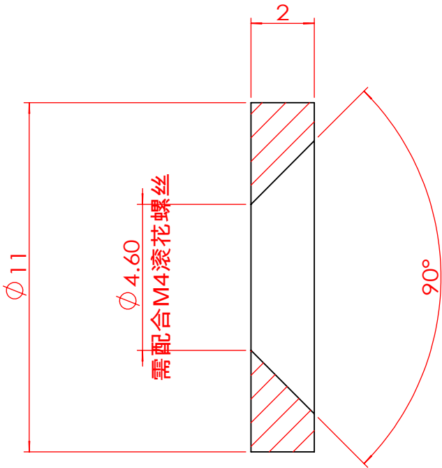
剖面 B-B
