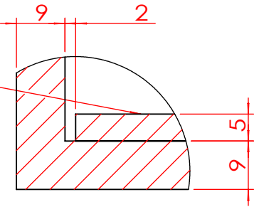
局部视图 C 比例 1 : 1
